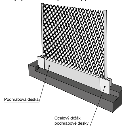
Plotový systém s ocelovými držáky podhrabové desky
