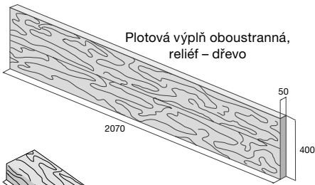
ZD plotové výplně, reliéf – dřevo
