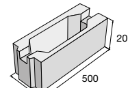
ZB 20-20
