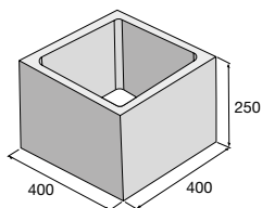
ST 40×40×25
