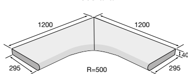
BL 120/30/4 VR S R 0,5 – vnitřní roh sestava
