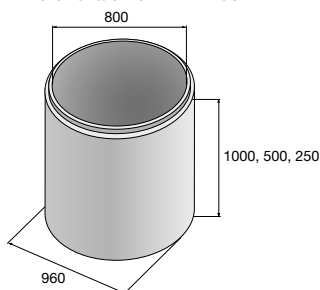
Betonová skruž TBX 2-80
