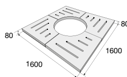
Stromová mříž – sestava 4 ks
