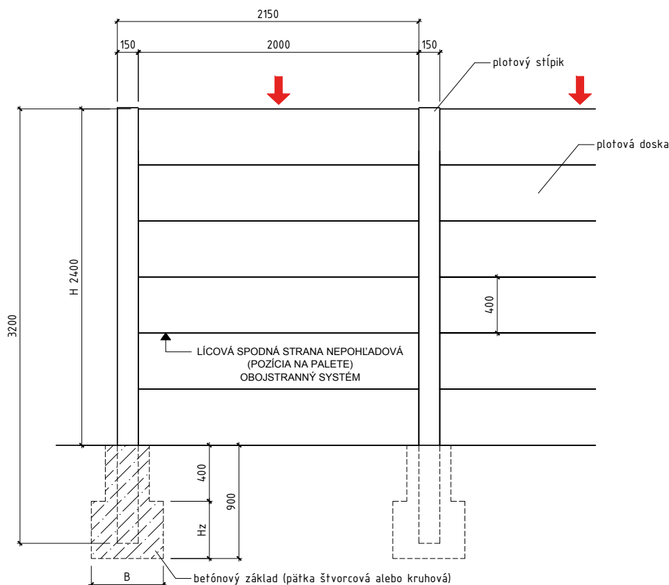
POHĽAD OPLOTENIA
