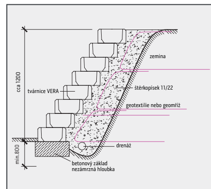
Schematický nákres uložení tvárnice VERA
