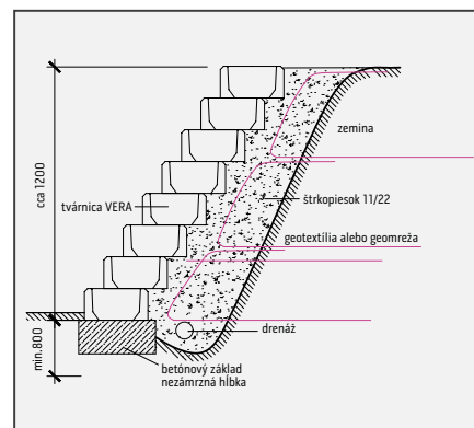
Schematický nákres uloženia tvárníc VERA
