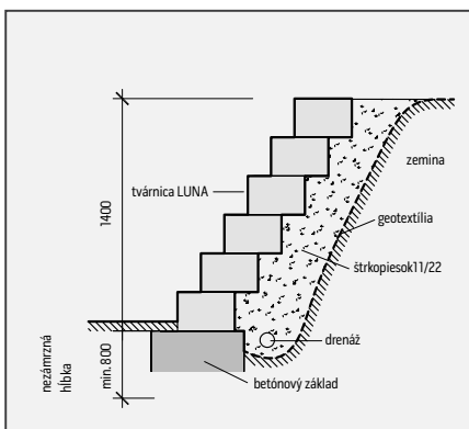
Schematický nákres uloženia tvárníc LUNA
