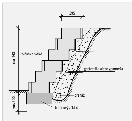
Schematický nákres uloženia tvárníc SÁRA
