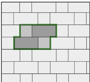
HOLLAND I – 33,33 ks / m 2 , 66,7 % dl. plochy HOLLAND II – 33,33 ks / m 2 , 33,3 % dl. plochy
