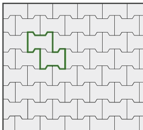
H-PROFIL – 35,35 ks /m 2 , 100 % dl. plochy
