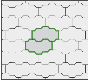
HYDROBAR – klasická skladba 39,7 ks / m 2 , 100 % dl. plochy
