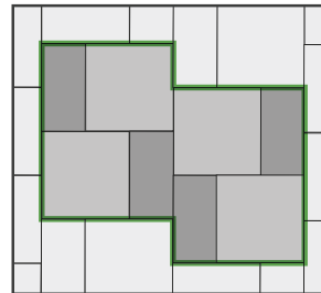
HOLLAND I – 16,67 ks / m 2 , 33,3 % dl. plochy HOLLAND III – 16,67 ks / m 2 , 66,7 % dl. plochy
