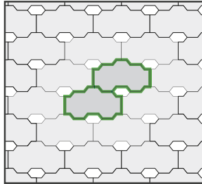
HYDROBAR – drenážní skladba 36,4 ks / m 2 , 91,7 % dl. plochy
