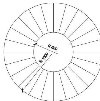
Klín BARK
