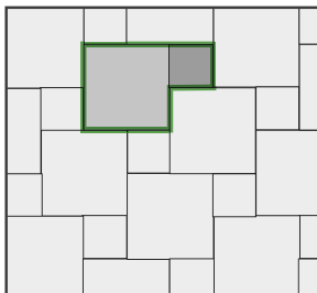
HOLLAND II – 20 ks / m 2 , 20 % dl. plochy HOLLAND III – 20 ks / m 2 , 80 % dl. plochy
