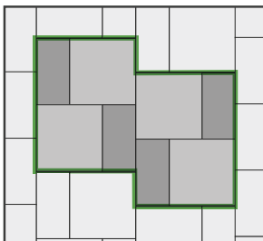
GRITO I – 16,67 ks / m 2 , 33,3 % dl. plochy GRITO III – 16,67 ks / m 2 , 66,7 % dl. plochy
