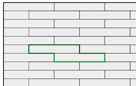
WOODY 3 - 4,17 ks/m 2 , 100% dl. plochy
