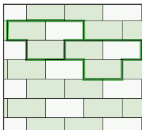
HOLLAND I světlá – 16,67 ks / m 2 , 33,3 % dl. plochy HOLLAND I tmavá – 33,33 ks / m 2 , 66,7 % dl. plochy
