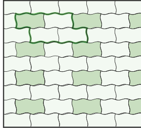
PAROLIN světlá – 26,04 ks / m 2 , 75 % dl. plochy PAROLIN tmavá – 8,68 ks / m 2 , 25 % dl. plochy
