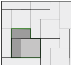
HOLLAND I – 25 ks / m 2 , 50 % dl. plochy HOLLAND III – 12,50 ks / m 2 , 50 % dl. plochy
