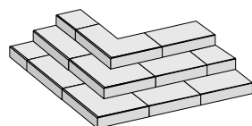
Rohový stupeň 90°
