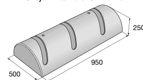
Koš TAMPA s oklepávátkem
