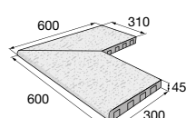
Bazénový lem VERTO – vnější roh
