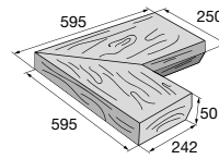
Bazénový lem BARK vnitřní roh
