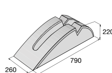
Stojan na kolo SK 1 – 1
