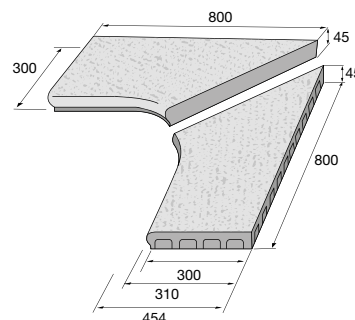
Bazénový lem VERTO – roh R 0,49 PUL pravá a levá
