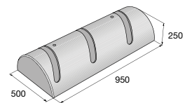
Stojan na kolo SK 2-3 str. 145
