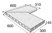
Bazénový lem VERTO – vnitřní roh
