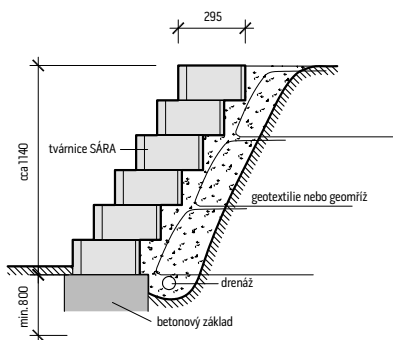
Schematický nákres uložení tvárnice SÁRA
