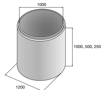
Betonová skruž TBX 2-100
