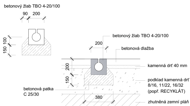
Schématiký příklad zabudování žlabů řady TBO 4-20/100.
