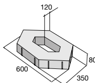
Vegetační dlažba H-E-X 120
