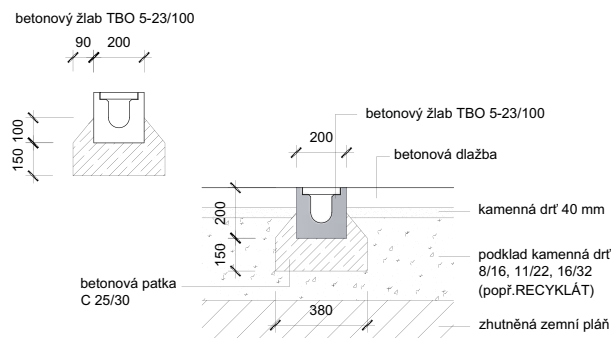
Schématiký příklad zabudování žlabů řady TBO 5-23/100.
