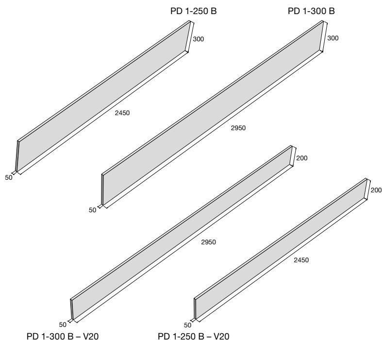
Plotová patka, podhrabová deska
