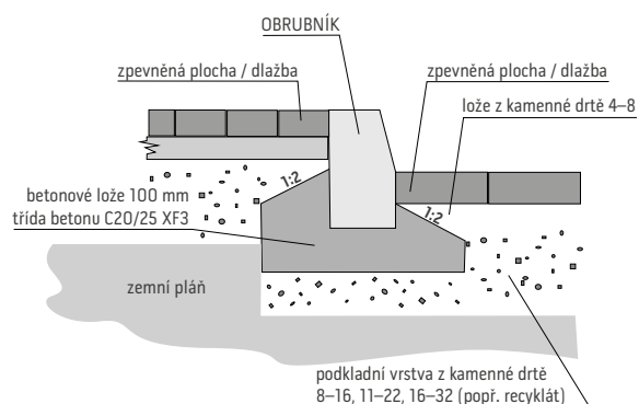
Schematické vyobrazení usazování obrubníku v dlážděné ploše
