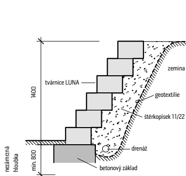
Schematický nákres uložení tvárnice LUNA
