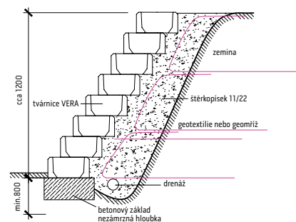
Schematický nákres uložení tvárnice VERA
