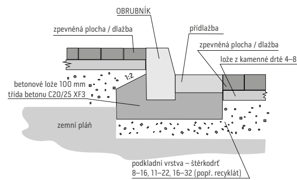
Schematické vyobrazení usazování obrubníku a přídlažby
