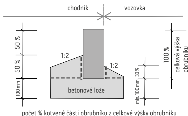
Základní schéma zabudování obrubníku
