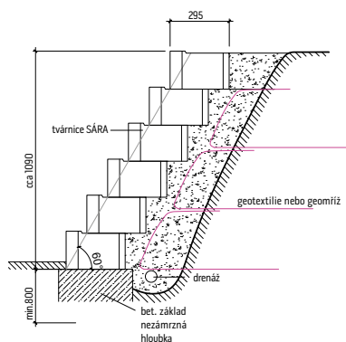
Schematický nákres uložení tvárnice SÁRA
