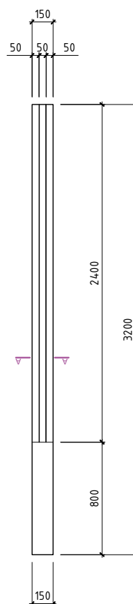
POHLED SLOUPEK DRÁŽKA
