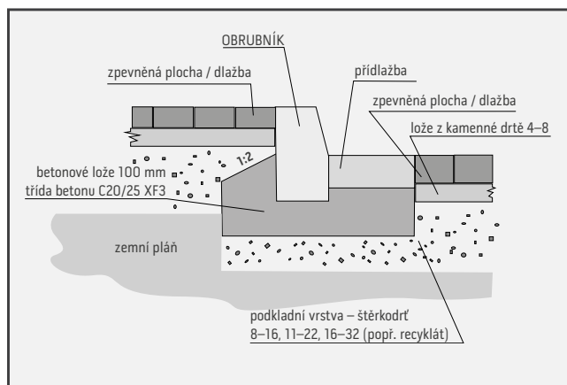
Schematické vyobrazení usazování obrubníku a přidlažby
