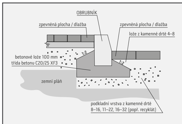
Schematické vyobrazenie usadzovania obrubníka v dlaždenej ploche
