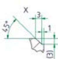
Detail fazety dlažba hr. 120 mm
