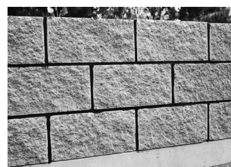
HOTOVÉ MURIVO: pri precíznom uzatvorení škár sú spoje odolné voči poveternostným vplyvom a mrazu a konštrukcia pôsobí po vyzrení výplňového betónu ako jeden monolitický celok.
