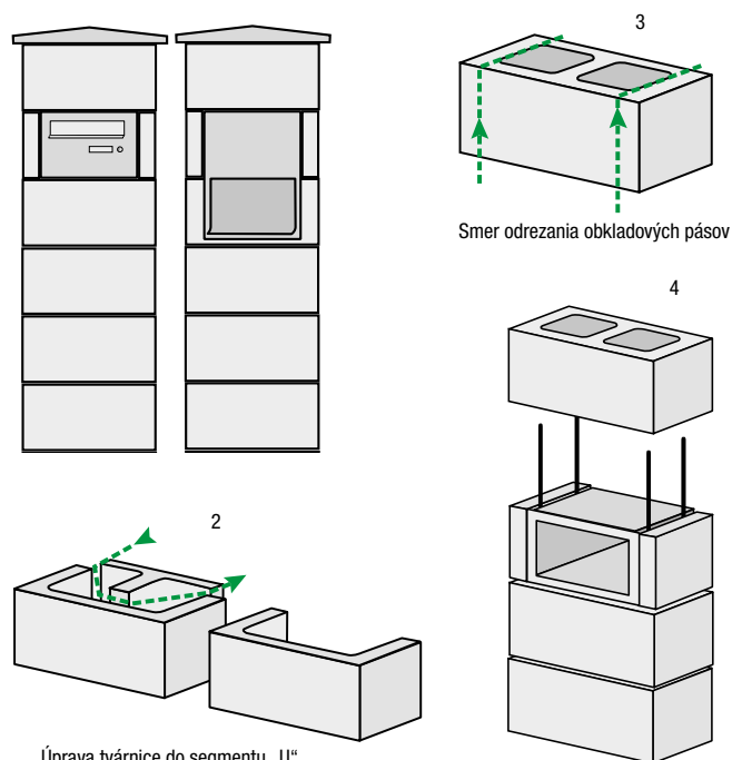
Úprava tvárnice do segmentu „U“
