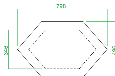
Pôdorys
