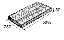
Dlažba OAK 3 N
